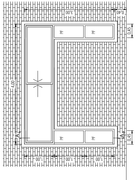
V3-RENOVACION VISTA
