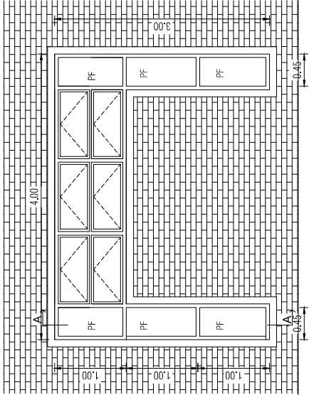
V3-EXISTENTE VISTA
