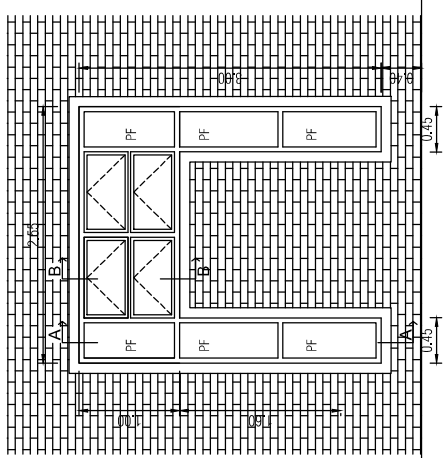
PLANTA
